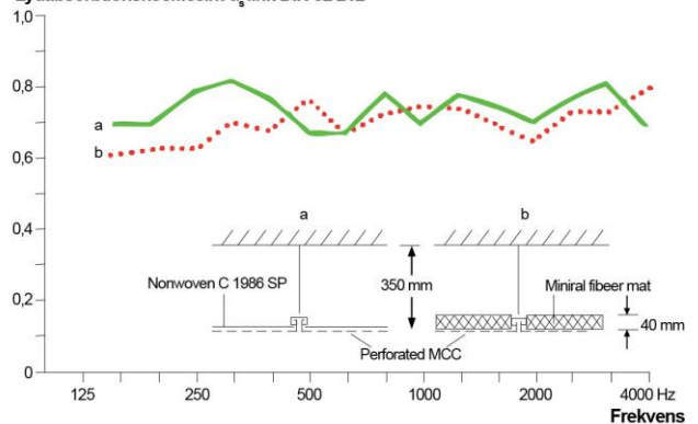
Lyddabsorptionskoefficient \alpha_s i.h.t DIN 52 212
